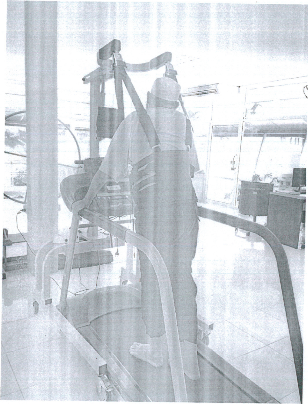
รูปที่ 7 ฝึกผู้ป่วยเดินด้วยเครื่อง litegait
